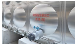
抗震型储水槽上设有紧急供水口，可在停水停电状态下确保居民有水可饮。
